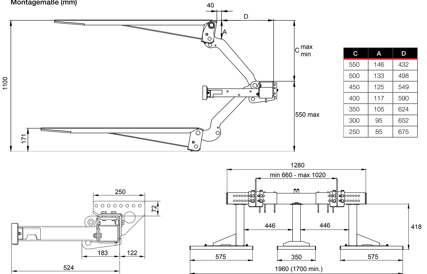
Montagemaße (mm)
