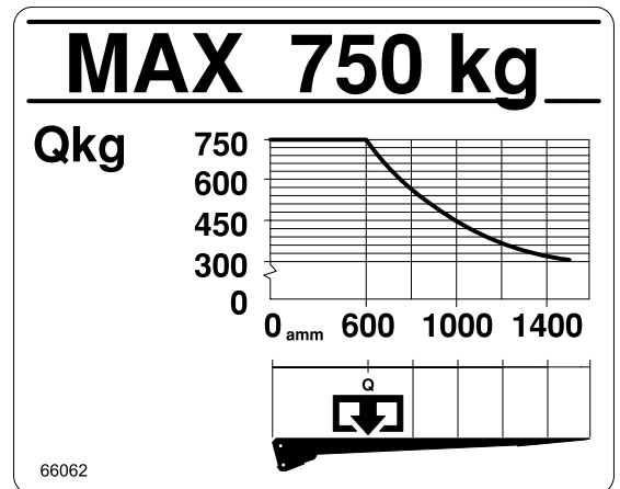
Belastningsdiagram
