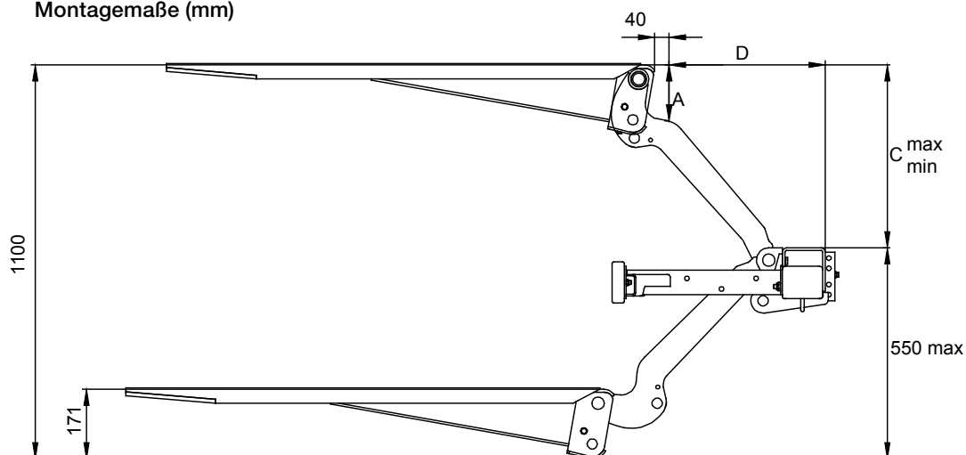
Montagemaße (mm)
