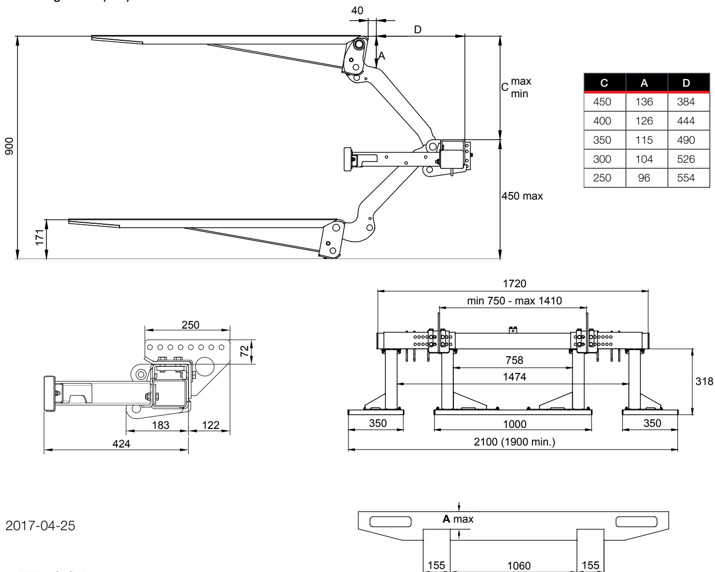
Montagemaße (mm)
