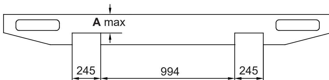
Bild 16. Urtag ur bakbalken
