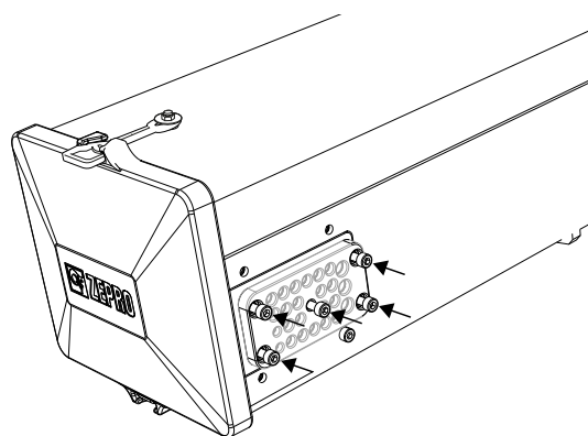
Bild 75. Kabelgenomföringens fem skruvar
