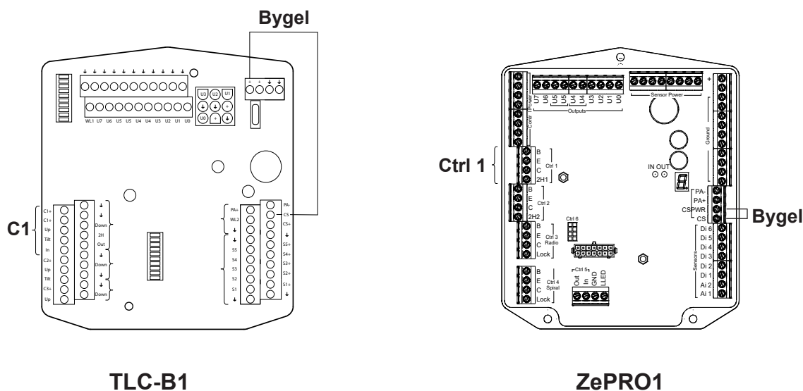
Bild 23. Tillfälligt inkoppling
