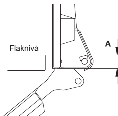
Bild 34. Kontrollera läget i förhållande till bilens bakbalk
