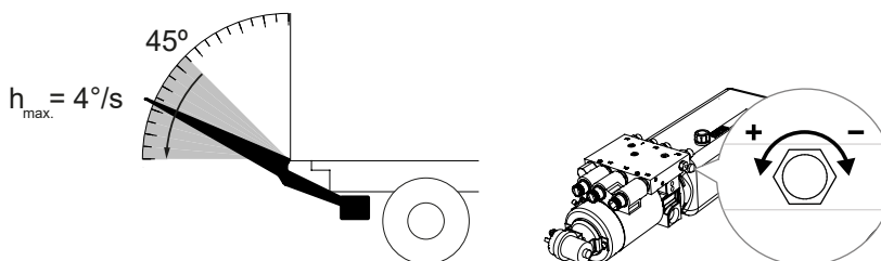
Bild 53. Inställning av tilthastighet nedåt inom arbetsområdet (från 45° och nedåt)
