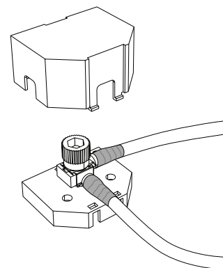
Bild 82. Skyddslock säkringslåda
