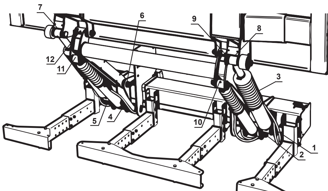
Bild 98. Smörjpunkter
