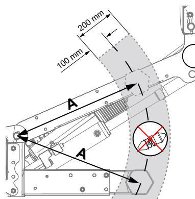
Bild 73. Placering av snabbkontakt
