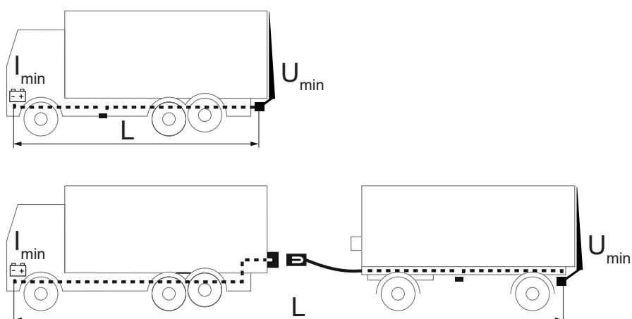
Bild 67. Maximal strömförbrukning - Minsta rekommenderade ledningsarea
