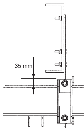
Bild 28. Ramfästet kräver minst 35 mm utrymme mellan fordonsram och lyftstomme
