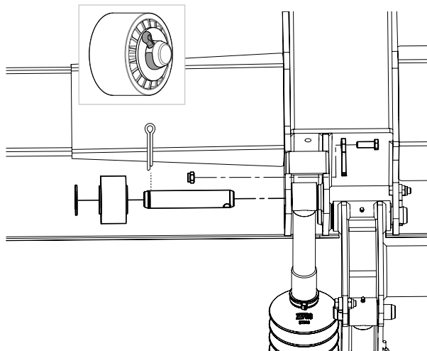
Bild 39. Montera tiltcylindern på plattformn
