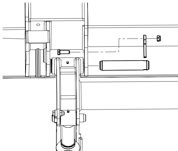
Bild 32. Montera plattformen på armarna
