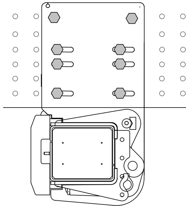
Bild 30. Montering av ramfästet på fordonsram med förborrade hål
