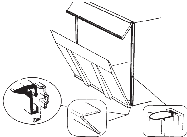
Bild 46. Montering av tättningslist
