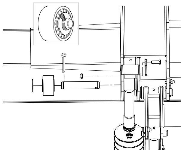
Bild 33. Montera tiltcyldern på plattformen
