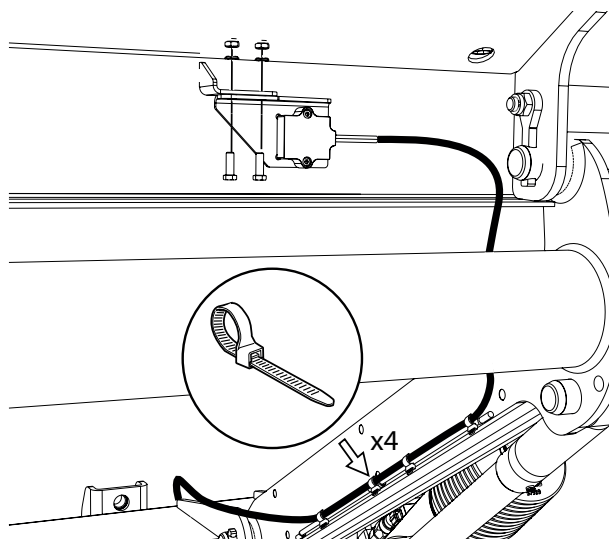
Bild 55. Montering Inklinometer
