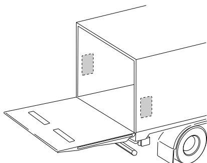
Bild 88. Standardmontering
