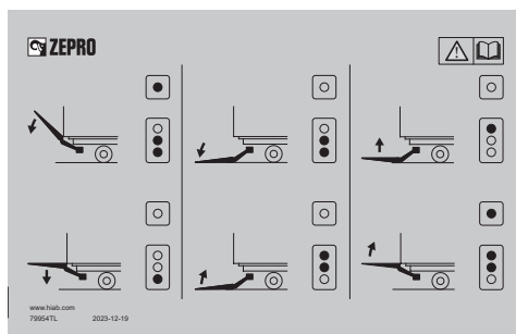
Bild 93. Manöverdonsdekal för CD 1 med tvåhandsknappen monterad ovanför manöverdonet.
