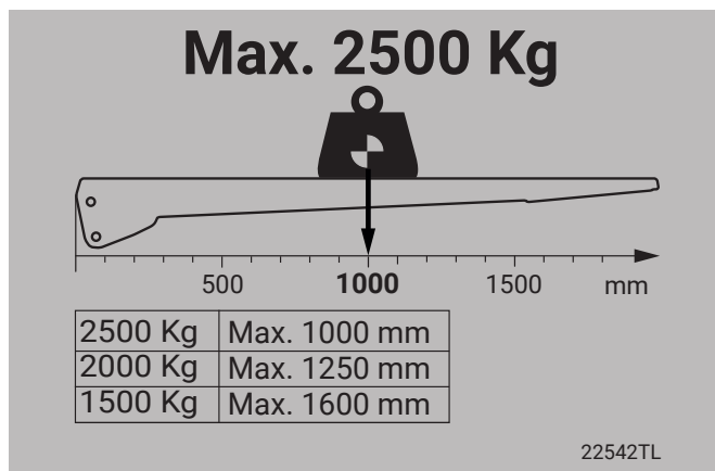
Bild 84. Belastningsdiagram för lastkapacitet 2500 Kg, tyngdpunktsavstånd 1000 mm.
