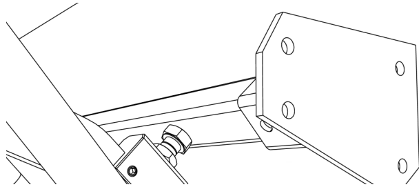
Bild 45. Montera anslagsklackar mellan lyftarmar och flakets bakbalk
