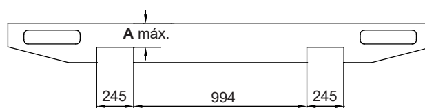
Imagen 18. Z 1500/2000
