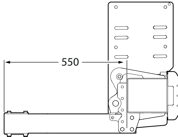
Imagen 14. Z 1500/2000 -135
