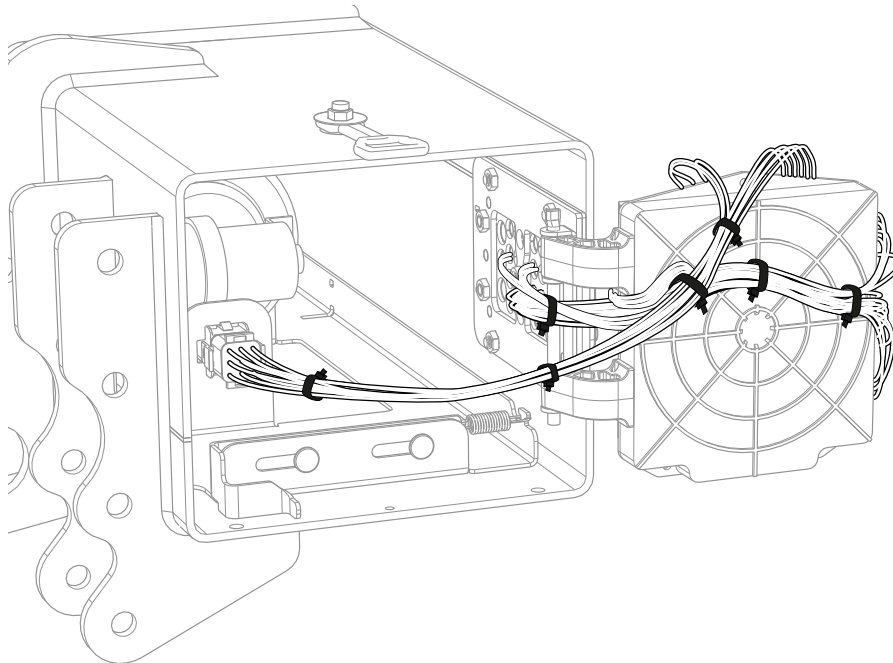
Imagen 79. Montaje del cableado con bridas
