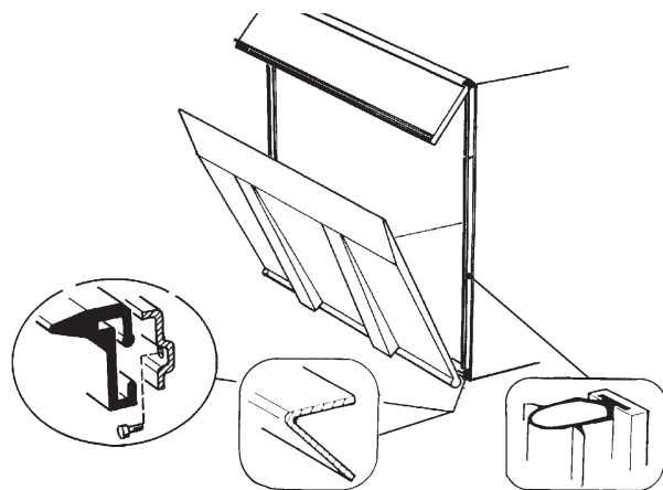
Imagen 48. Montaje del listón de sellado
