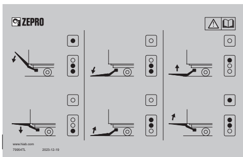
Imagen 97. Etiqueta del dispositivo de mando para CD 1 con el botón de dos manos montado encima del dispositivo de mando.
