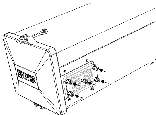
Imagen 77. Los cinco tornillos del prensaestopas
