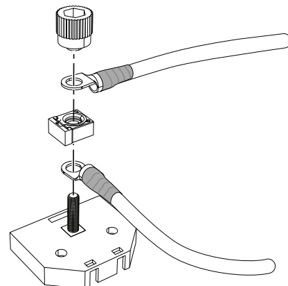
Imagen 71. Conexión a la caja de fusibles
