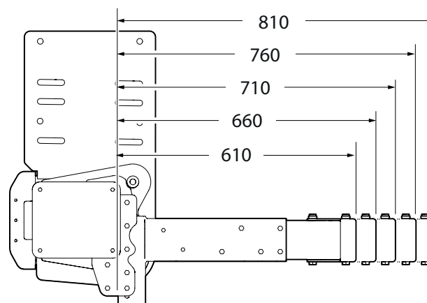
Imagen 50. La parte exterior de los soportes se puede montar en cuatro posiciones diferentes
