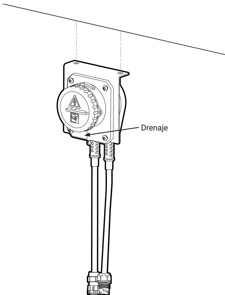
Imagen 72. Montaje del interruptor principal
