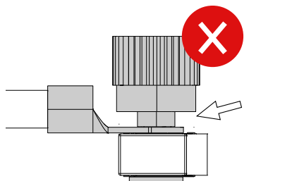
Imagen 83. Montaje incorrecto
