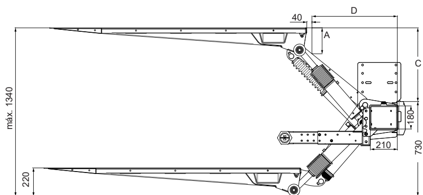
Imagen 11. Z 1500/2000-135
