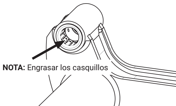
Imagen 33. Asegurarse de lubricar inicialmente los casquillos metálicos
