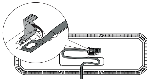
Imagen 62. Desconexión del contacto
