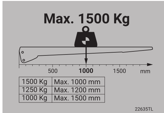
Imagen 87. Diagrama de carga para una capacidad de carga de 1500 kg, distancia al centro de gravedad 1000 mm.
