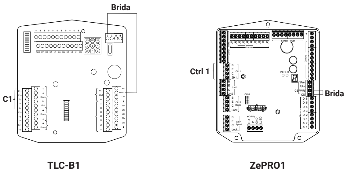
Imagen 25. Conexión temporal
