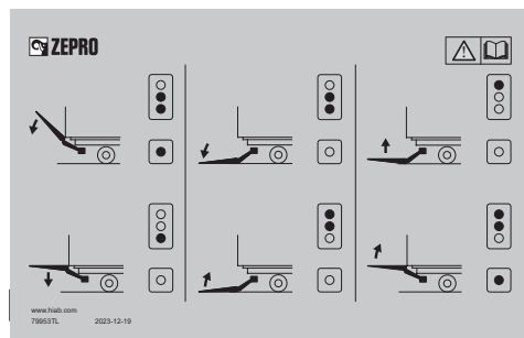
Imagen 98. Etiqueta del dispositivo de mando para CD 1 con el botón de dos manos montado debajo del dispositivo de mando.
