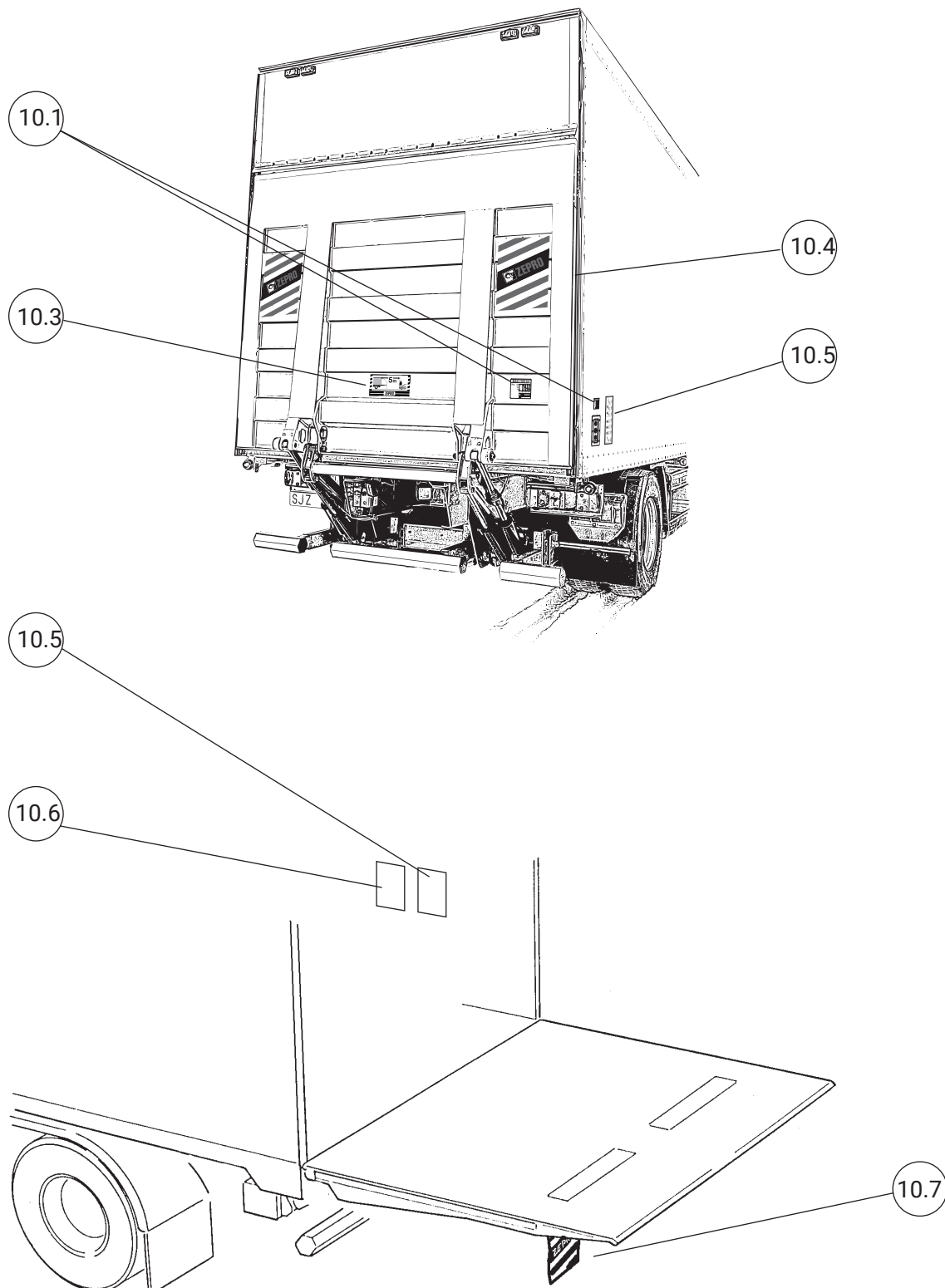
Imagen 86. Visión de conjunto del marcado
