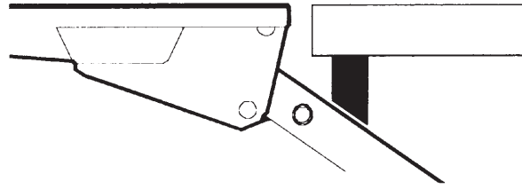
Imagen 47. Montar tacos de tope entre los brazos de elevación y la barra trasera de la plataforma
