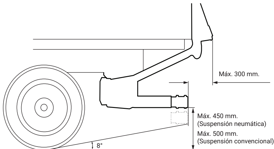
Imagen 8. Medidas reglamentarias
