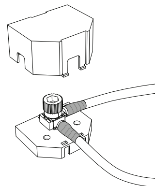
Imagen 84. Tapa protectora de la caja de fusibles
