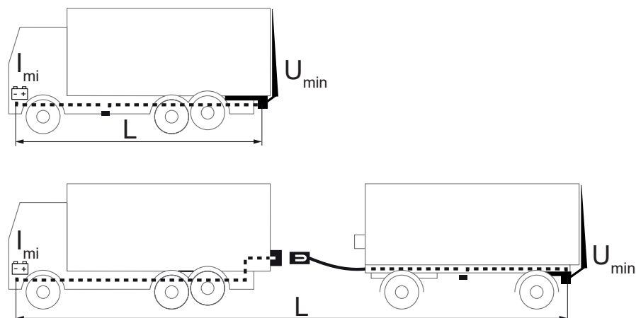
Imagen 69. Capacidad de la batería y definición de la longitud del cable de conexión a tierra y de alimentación principal
