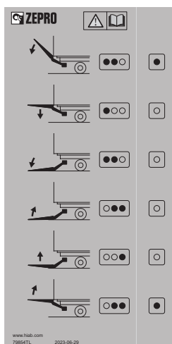
Imagen 99. La etiqueta del dispositivo de mando para CD 1, 2 y 9 para dispositivos de mando horizontales se encarga por separado. 79854TL
