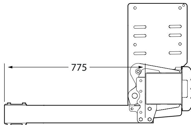
Imagen 16. Z 1500/2000 -175
