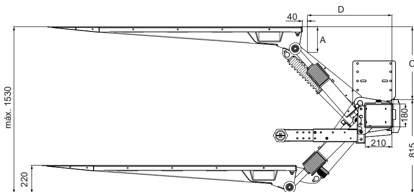
Imagen 12. Z 1500/2000-155
