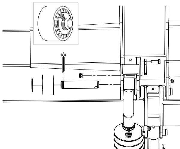
Imagen 35. Montar el cilindro de basculamiento en la plataforma
