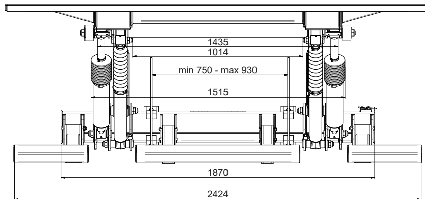
Imagen 17. Z 1500/2000
