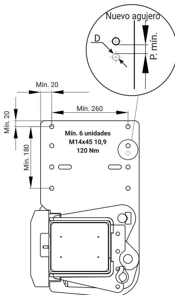
Imagen 31. Montar el soporte del chasis con 6 tornillos M14x45 10.9 como mínimo
