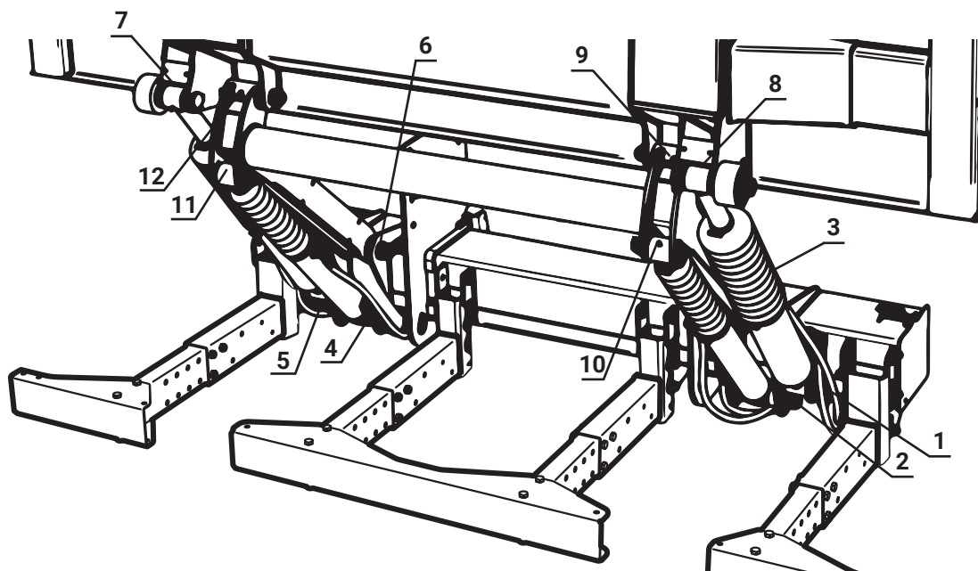
Imagen 85. Puntos de lubricación
