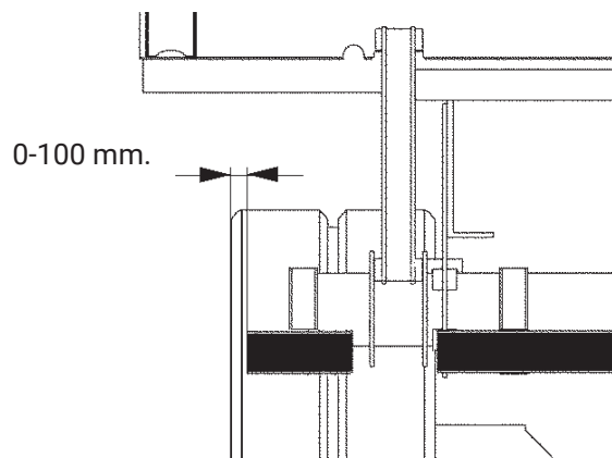
Imagen 9. Medidas reglamentarias
