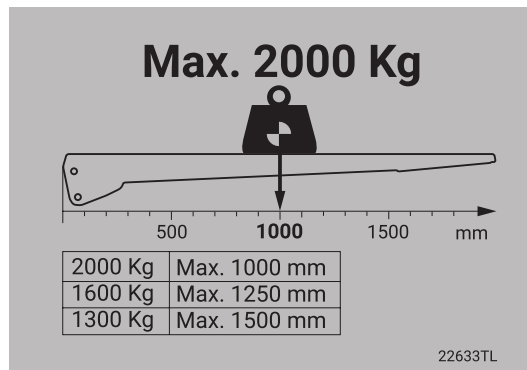
Imagen 88. Diagrama de carga para una capacidad de carga de 2000 kg, distancia al centro de gravedad 1000 mm.
