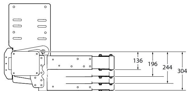
Imagen 49. La parte interior de los soportes se puede montar en cuatro alturas diferentes
