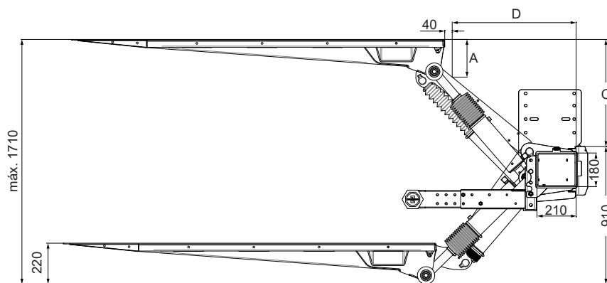
Imagen 13. Z 1500/2000-175
