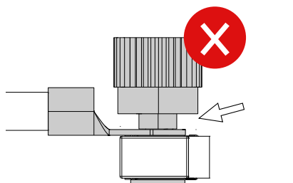
Bild 67. Felaktig montering
