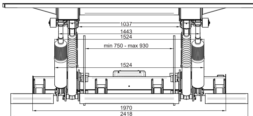
Bild 12. Inbyggnadsmått ZHD 3000-150
