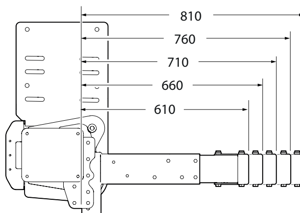
Bild 40. De yttre delen av konsolerna kan monteras i fem olika lägen
