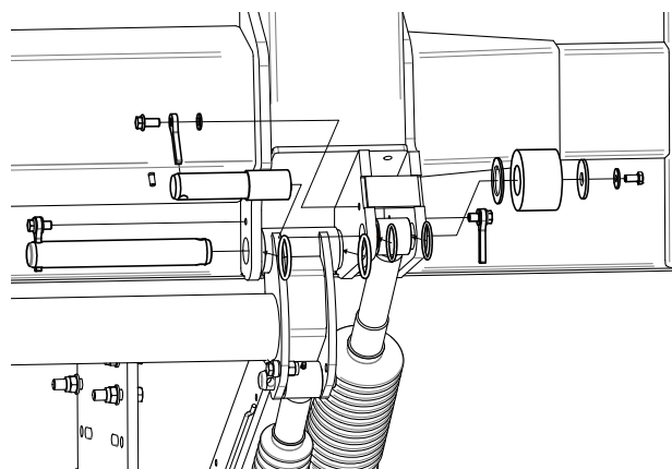
Bild 31. Montera den andra tilt-cylindern på plattformen
