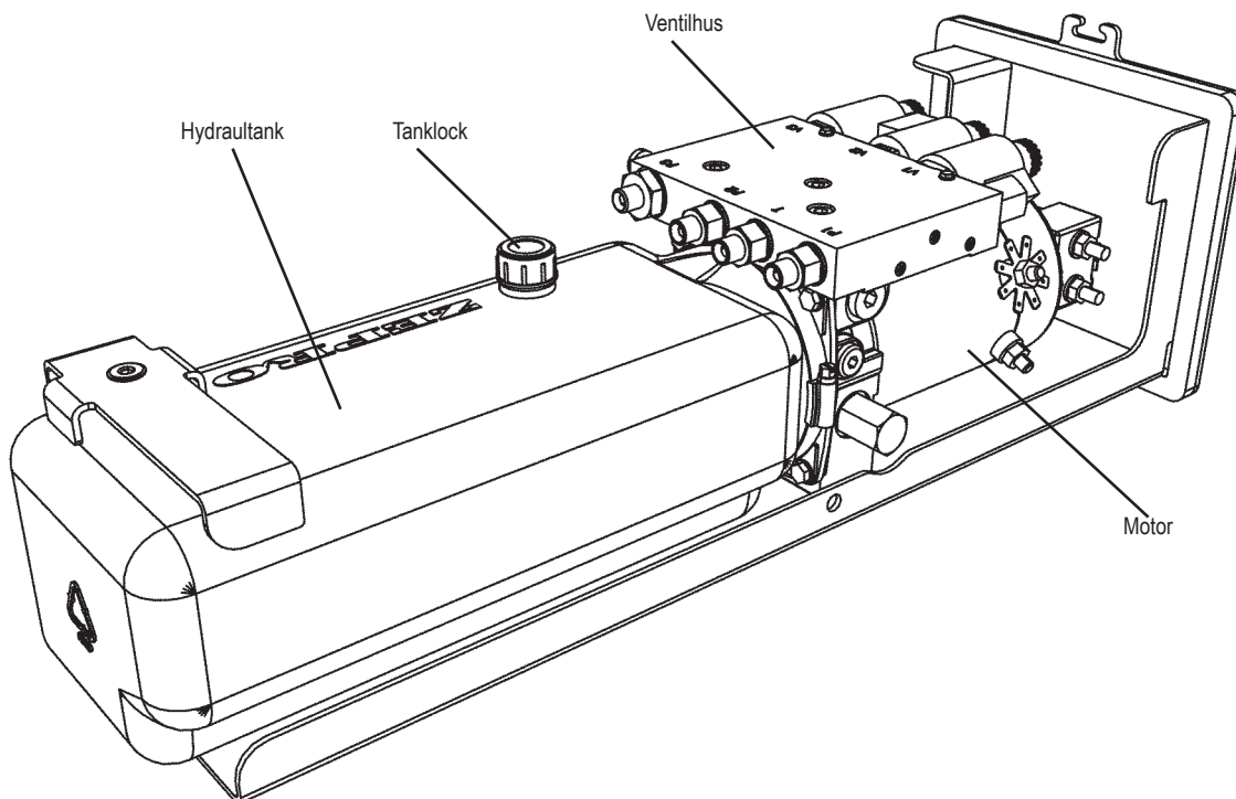
Bild 16. Hydraulaggregat
