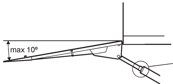
Bild 34. Nedtiltningsvinkel ska justeras till max 10°
