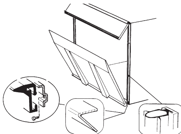
Bild 38. Montering av tätningslist
