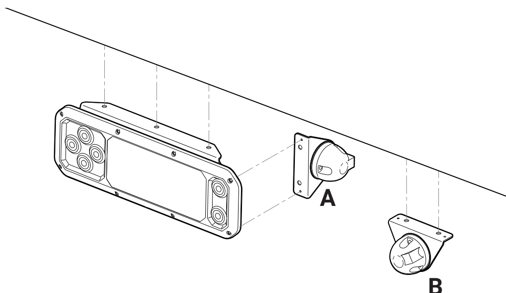
Bild 53. Montering av manöverdon CD19 och kontakt för handhållet manöverdon
