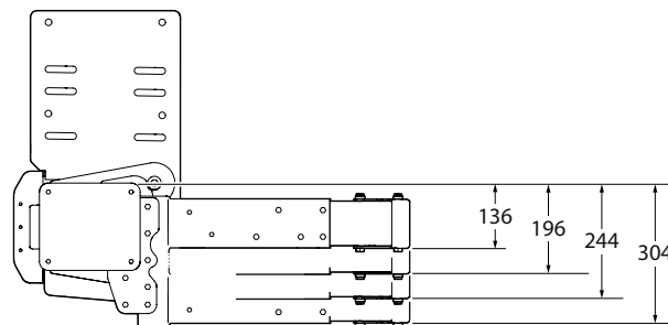
Bild 39. Den inre delen av konsolerna kan monteras i fyra olika höjdlägen
