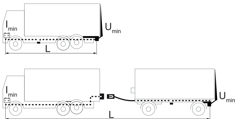
Bild 56. Batterikapacitet och definition av jord- och huvudströmkabels längd
