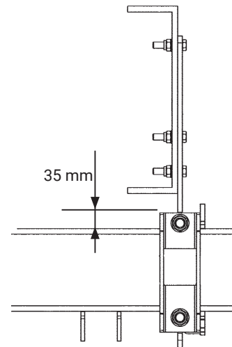
Bild 22. Ramfästet kräver minst 35 mm utrymme mellan fordonsram och lyftstomme
