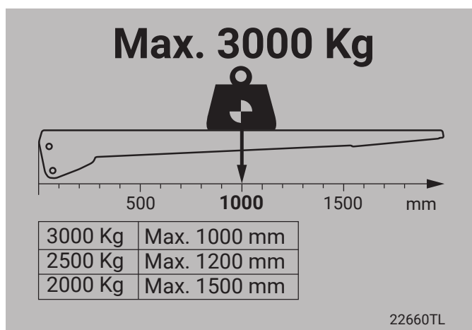
Bild 71. Belastningsdiagram för lastkapacitet 3000 Kg, tyngdpunktsavstånd 1000 mm.
