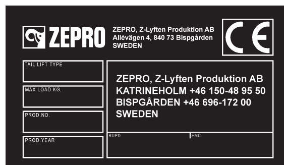
Bild 72. Typskylt
