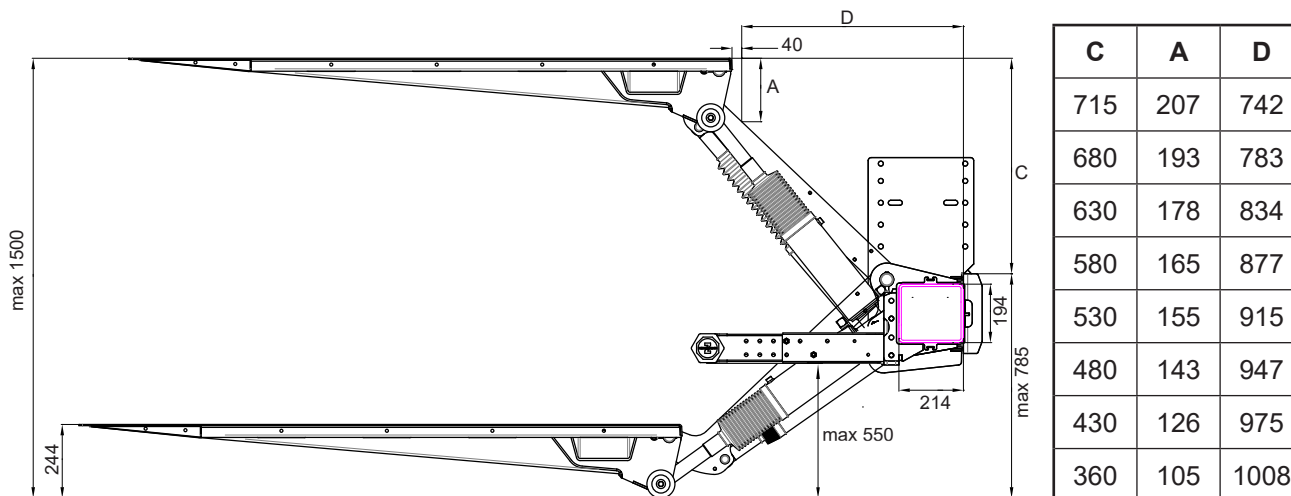
Bild 11. Inbyggnadsmått. Man bör sträva efter att sätta lyften så högt som möjligt inom angivna C-mått i tabellen.
