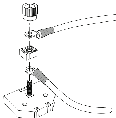
Bild 58. Inkoppling till säkringslåda
