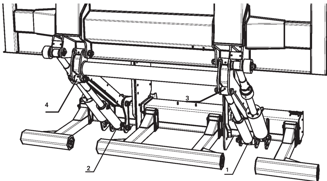
Bild 69. Smörjpunkter
