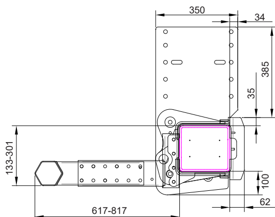
Bild 13. Ramfästets mått
