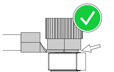
Bild 66. Korrekt montering
