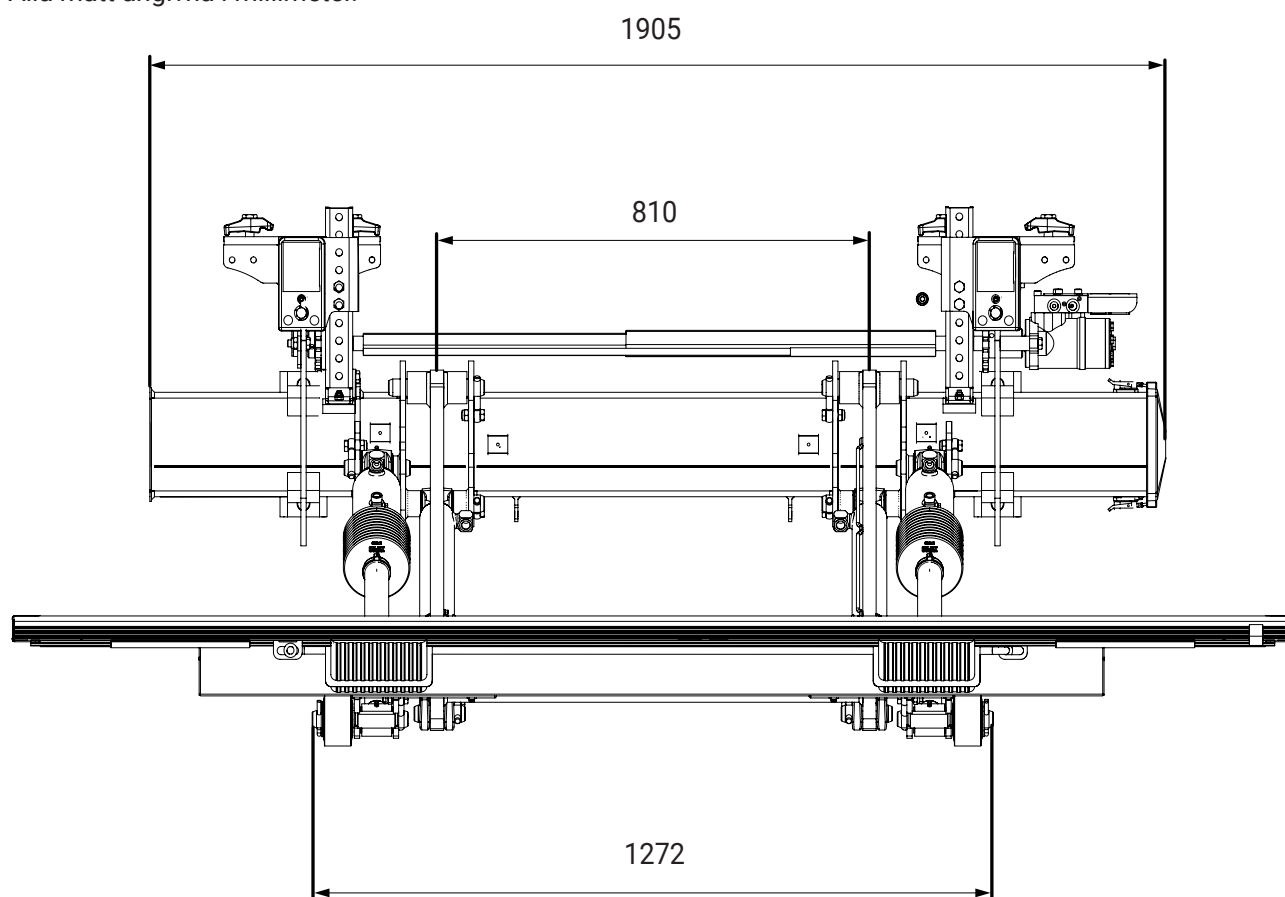
Bild 14. Inbyggnadsmått
