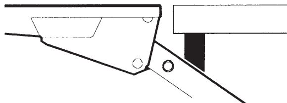
Bild 36. Montera anslagsklackar mellan lyftarmar och flakets bakbalk
