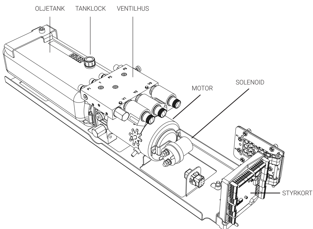
Bild 22. Hydraulaggregat och styrkort
