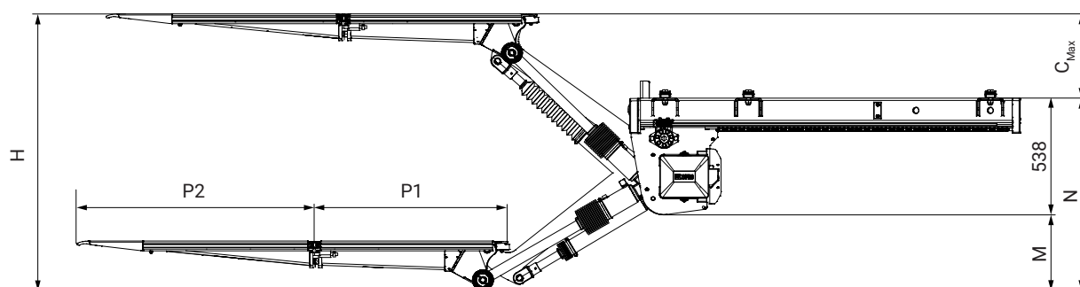
Bild 10. Inbyggnadsmått
