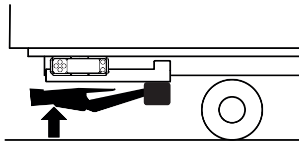
Bild 41. Montering av manöverdon
