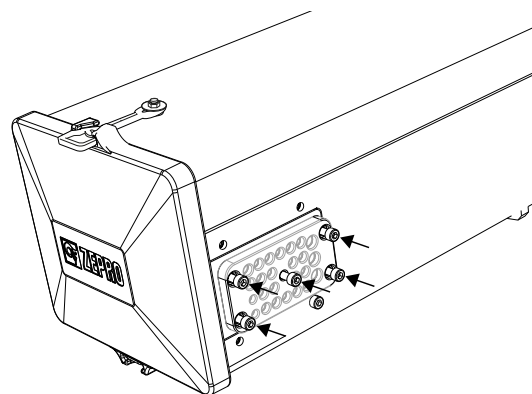
Bild 61. Kabelgenomföringens fem skruvar
