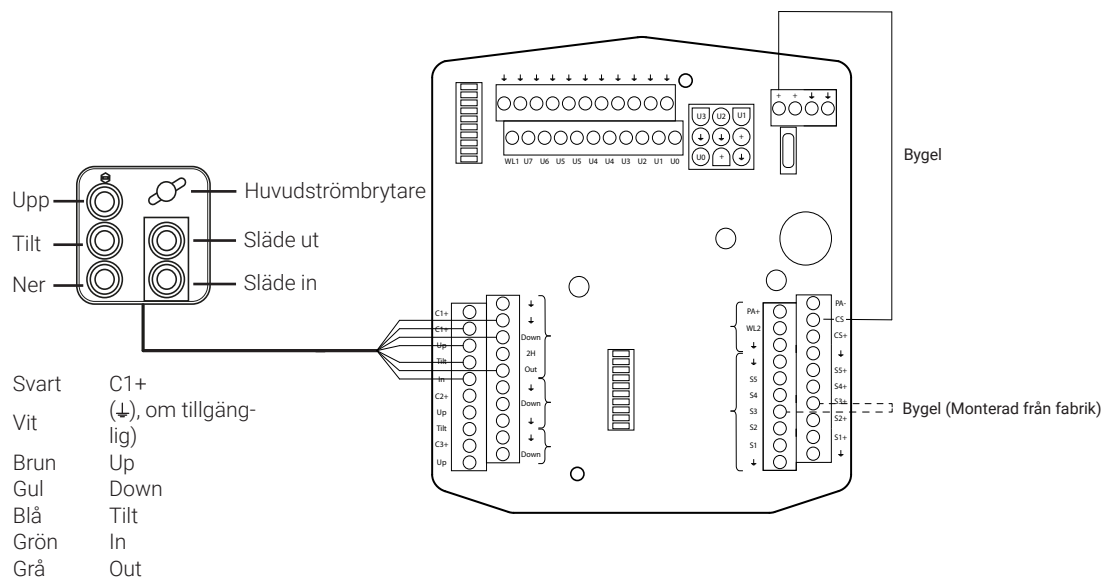
Bild 23. Tillfälligt inkoppling av manöverdon
