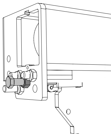
Bild 27. Skruv för inställning av arbetsposition
