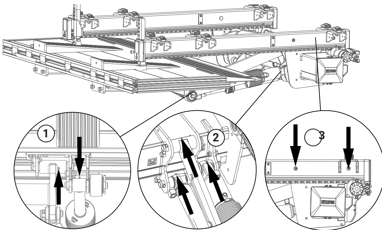
Bild 70. Smörjpunkter
