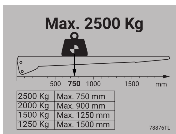
Bild 74. Belastningsdiagram för lastkapacitet 2500 Kg, tyngdpunktsavstånd 750 mm.
