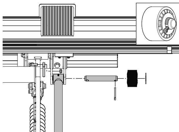
Bild 34. Montera tiltcylindern på bryggan
