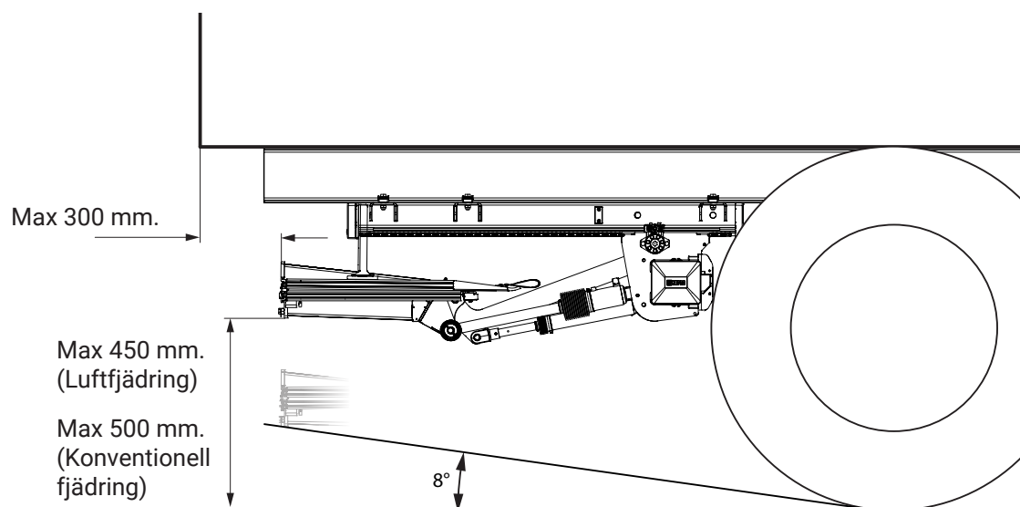
Bild 8. Lagstadgade mått för underkörningsskydd
