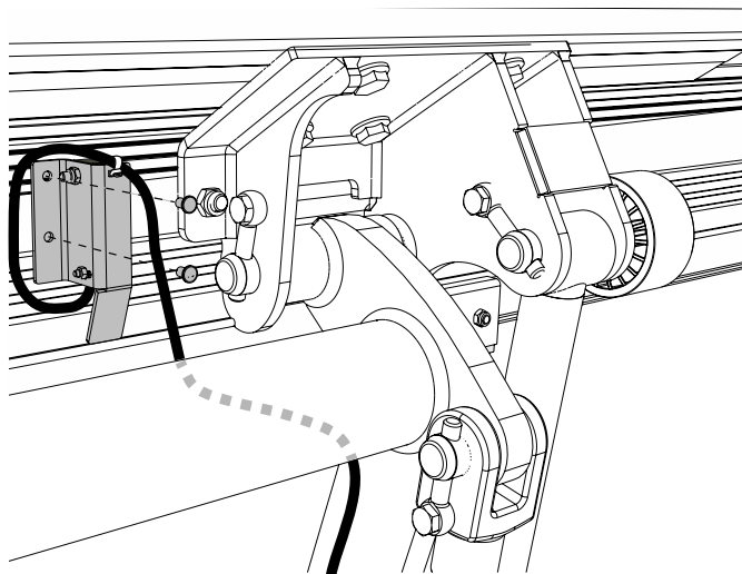
Bild 39. Montering av vinkelgivare
