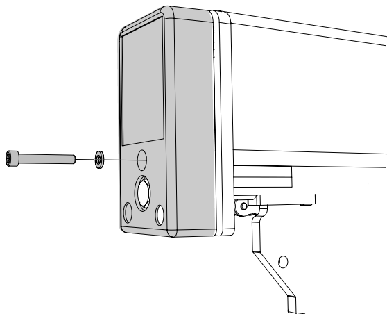
Bild 26. Slädprofilens ändkåpa
