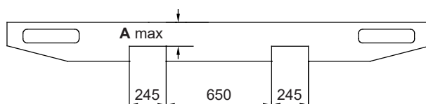
Bild 16. Urtag ur bakbalken
