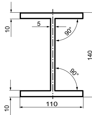
Bild 7. Tvärsnitt på fordonschassits rambalk (Alla mått angivna i millimeter)
