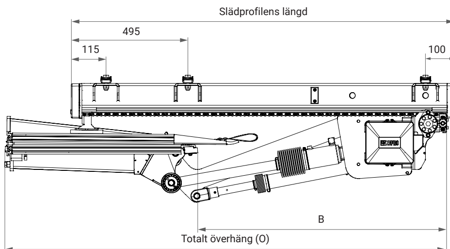
Bild 12. Inbyggnadsmått
