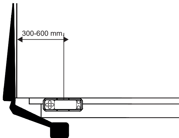
Bild 51. Montering av manöverdon
