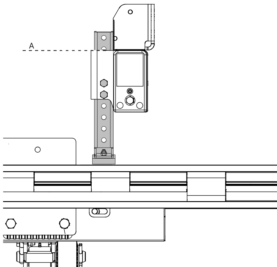
Bild 37. Montering av transportstoppen
