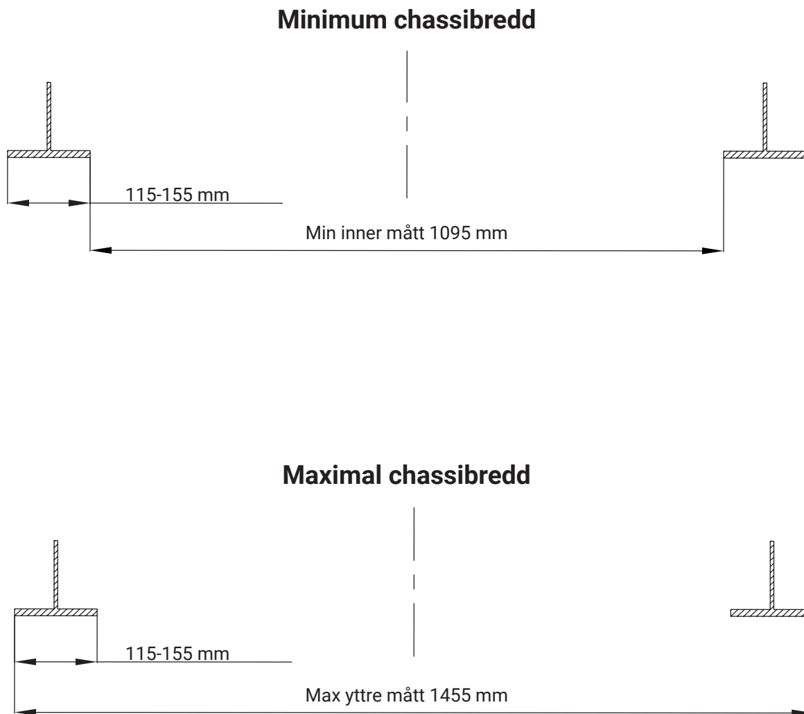
Bild 15. Rambredd, min- och maxmått
