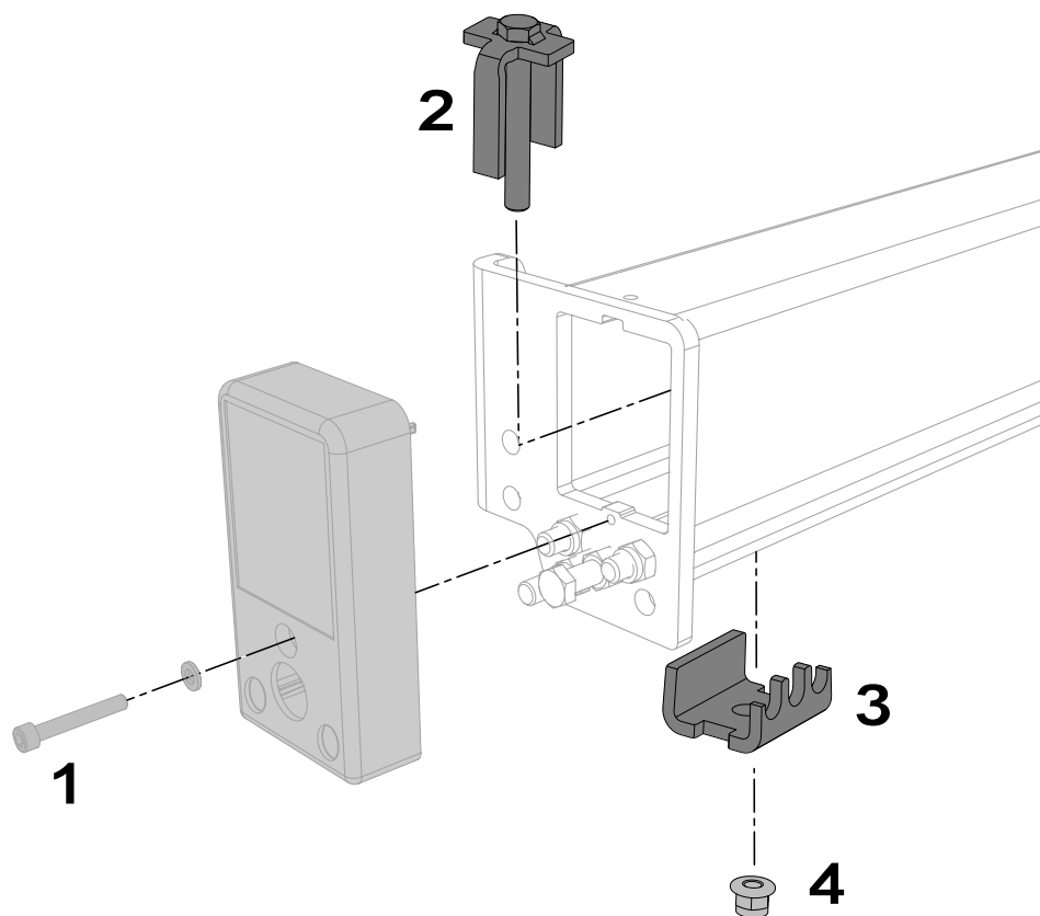
Bild 28. Arbetspositionsås (Tillval)
