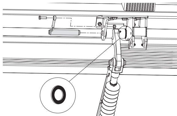
Bild 30. Montera lyftbryggan på armarna
