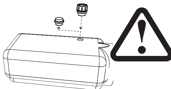
Bild 21. Ersätt transportpluggen med ordinarie tanklock
