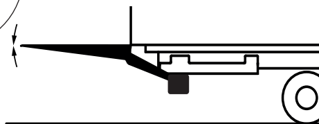
Bild 40. Justering av autotilt-vinkel
