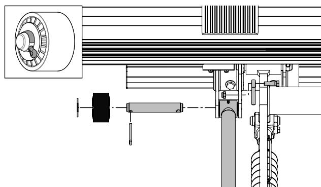
Bild 31. Montera tiltcyldern på bryggan
