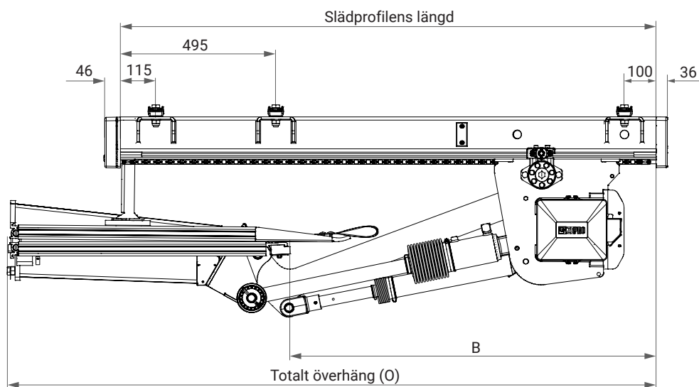
Bild 9. Inbyggnadsmått
