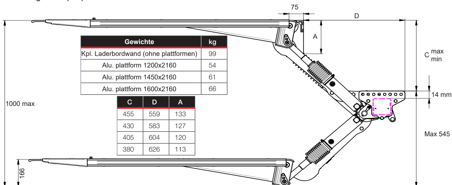
Montagemaße (mm)
