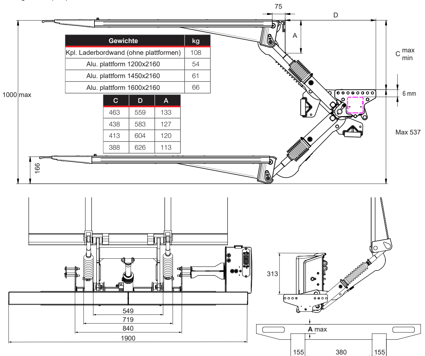
Montagemaße (mm)
