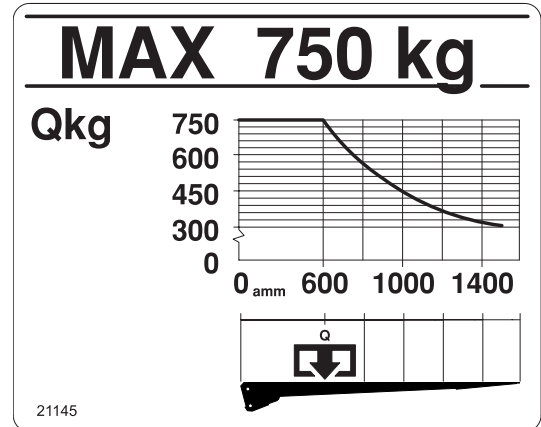
Belastungsdiagramm
