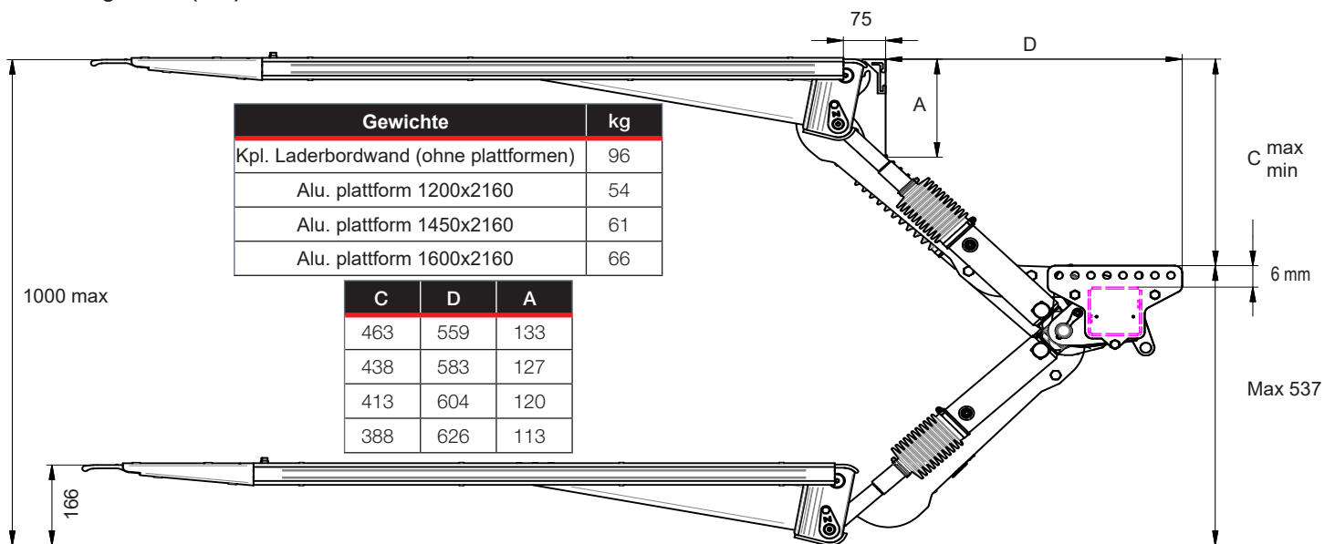
Montagemaße (mm)
